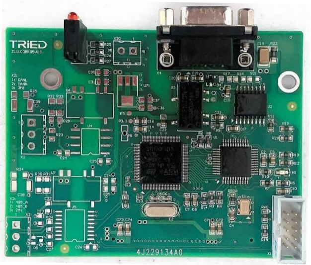
图 8.5 DP 通讯板
