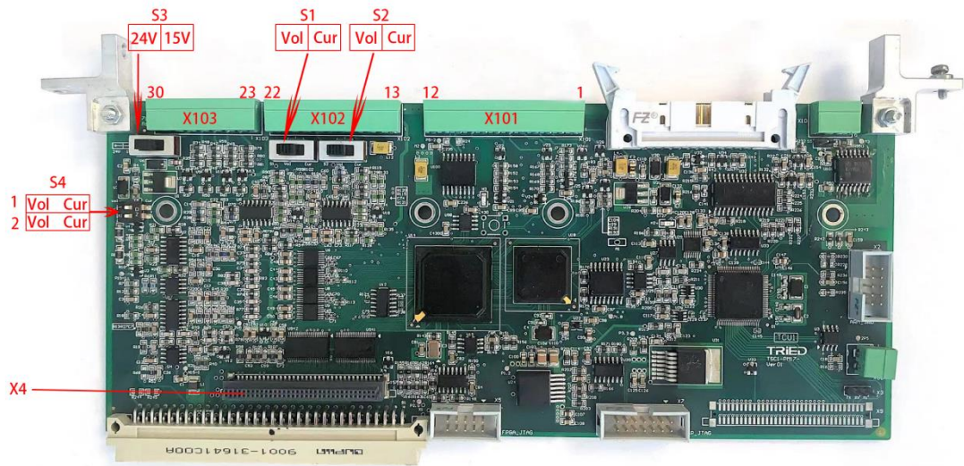
图 3.1 TAC1 系列工程型变频器的控制器 TCU1
